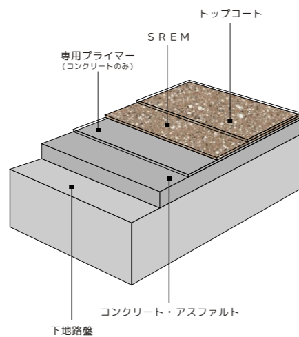
《SREMシリーズ御影石風 断面図》
